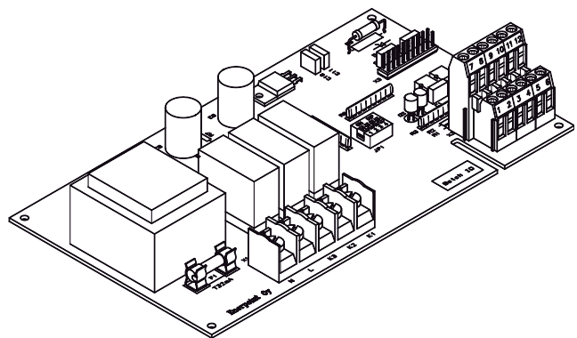
C260VKK Alakortti/Nedre kort, WX216
