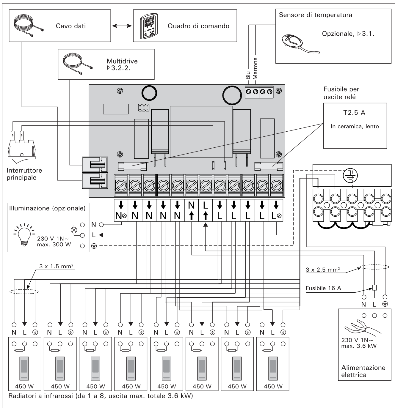
Figura 7. Collegamenti elettrici
