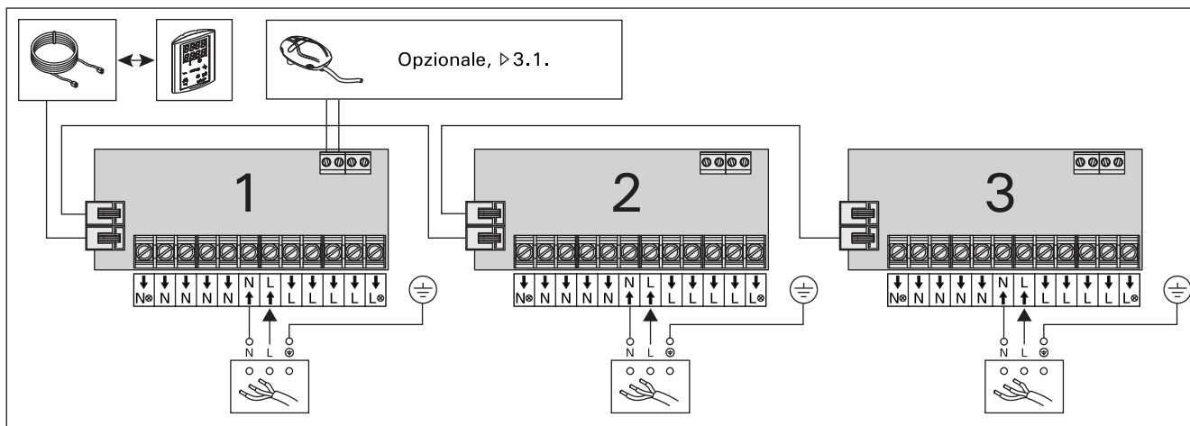
Figura 8. Serie di unità di alimentazione (Multidrive)
